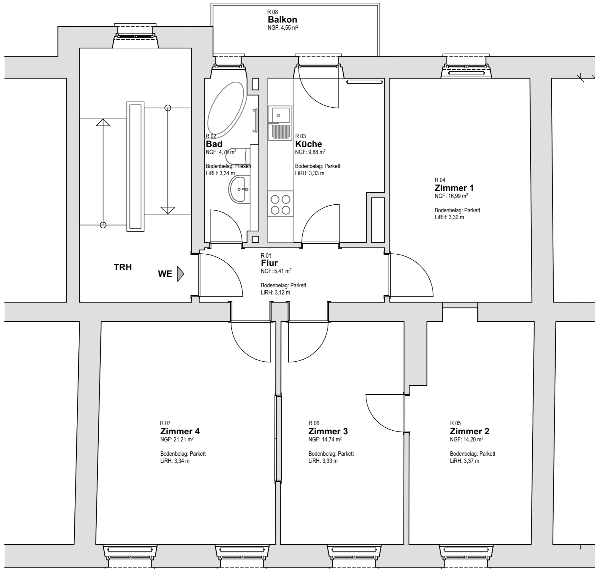
Grundriss
