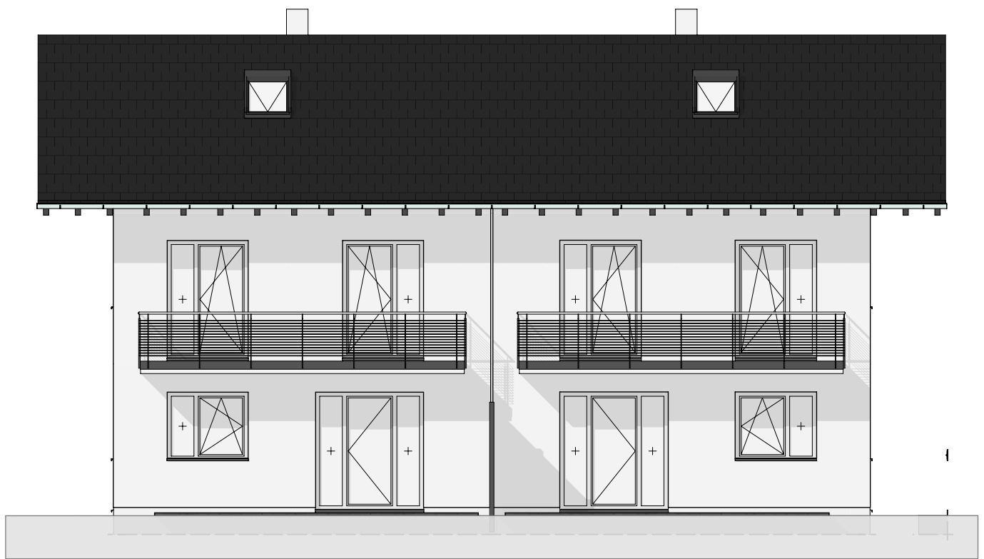
Ansicht Süd
