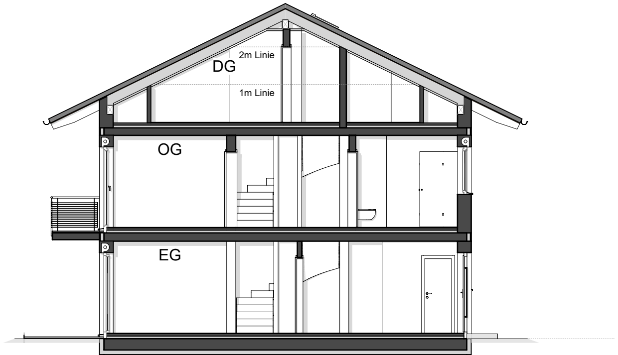
Schnitt A-A (Haus A)
