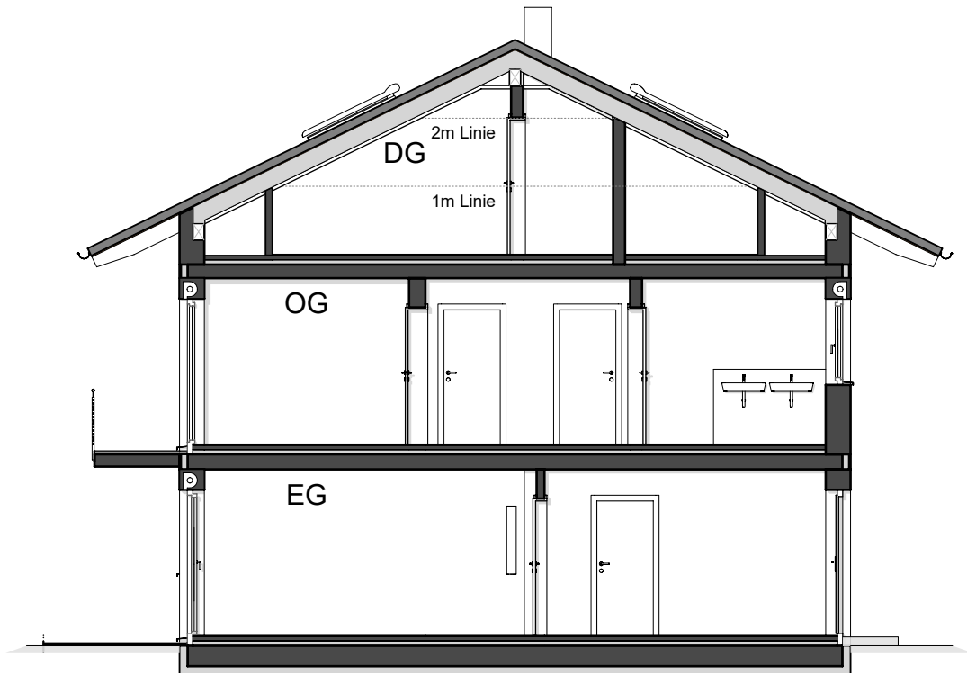
Schnitt B-B (Haus B)
