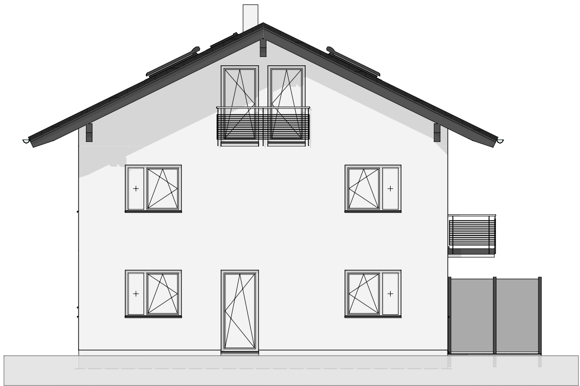
Ansicht West
