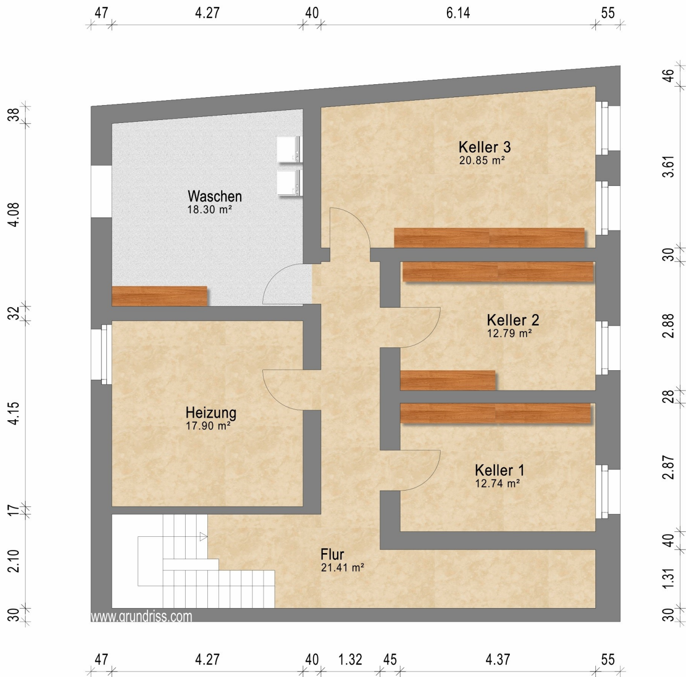
Kellergeschoss
