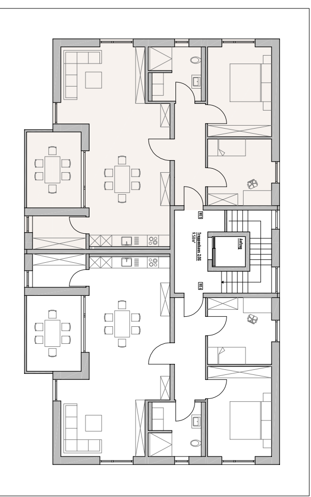
2. Obergeschoss
