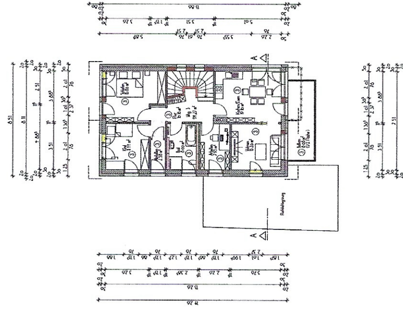
Grundriss Obergeschoss
