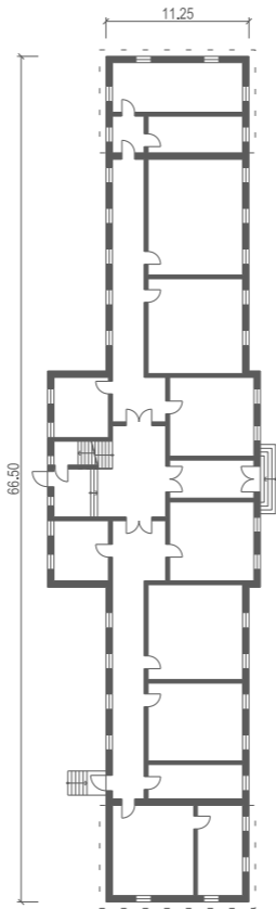
Grundriss EG
