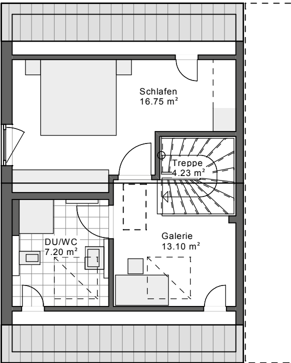
2,5 Geschosse Satteldach 38° ohne Kniestock
