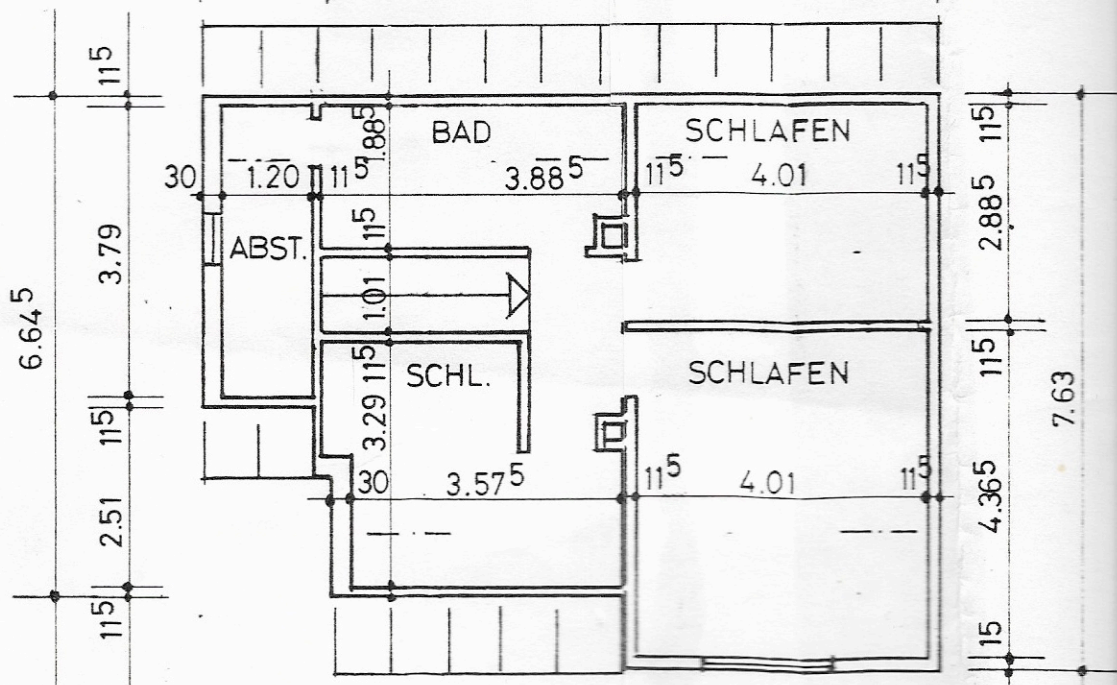
GRUNDRISS E.G.
