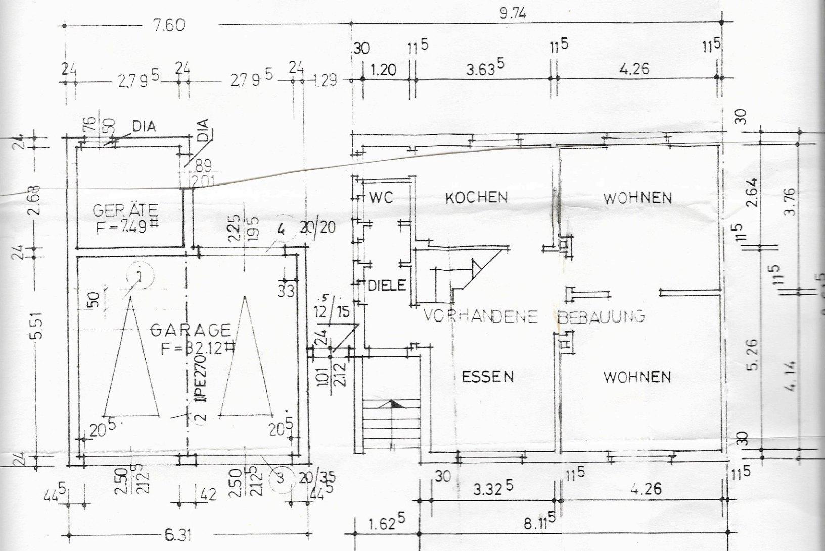
GRUNDRISS E.G.
