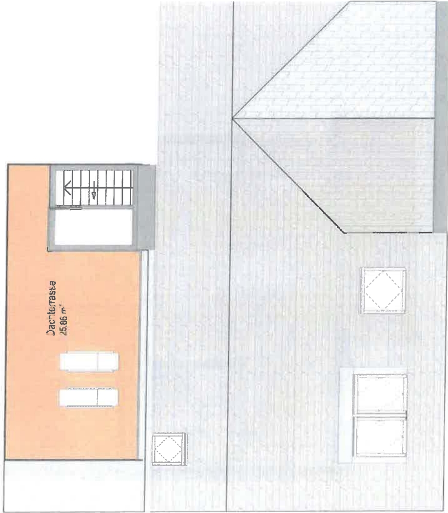
Grundriss Dachterrasse Top 11 M 1:100
