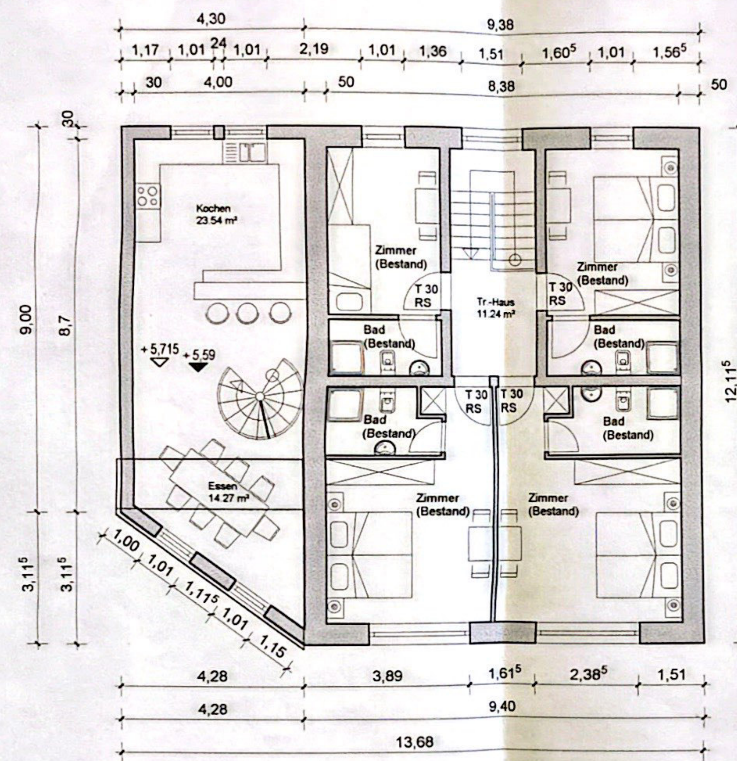
2. OBERGESCHOSS
