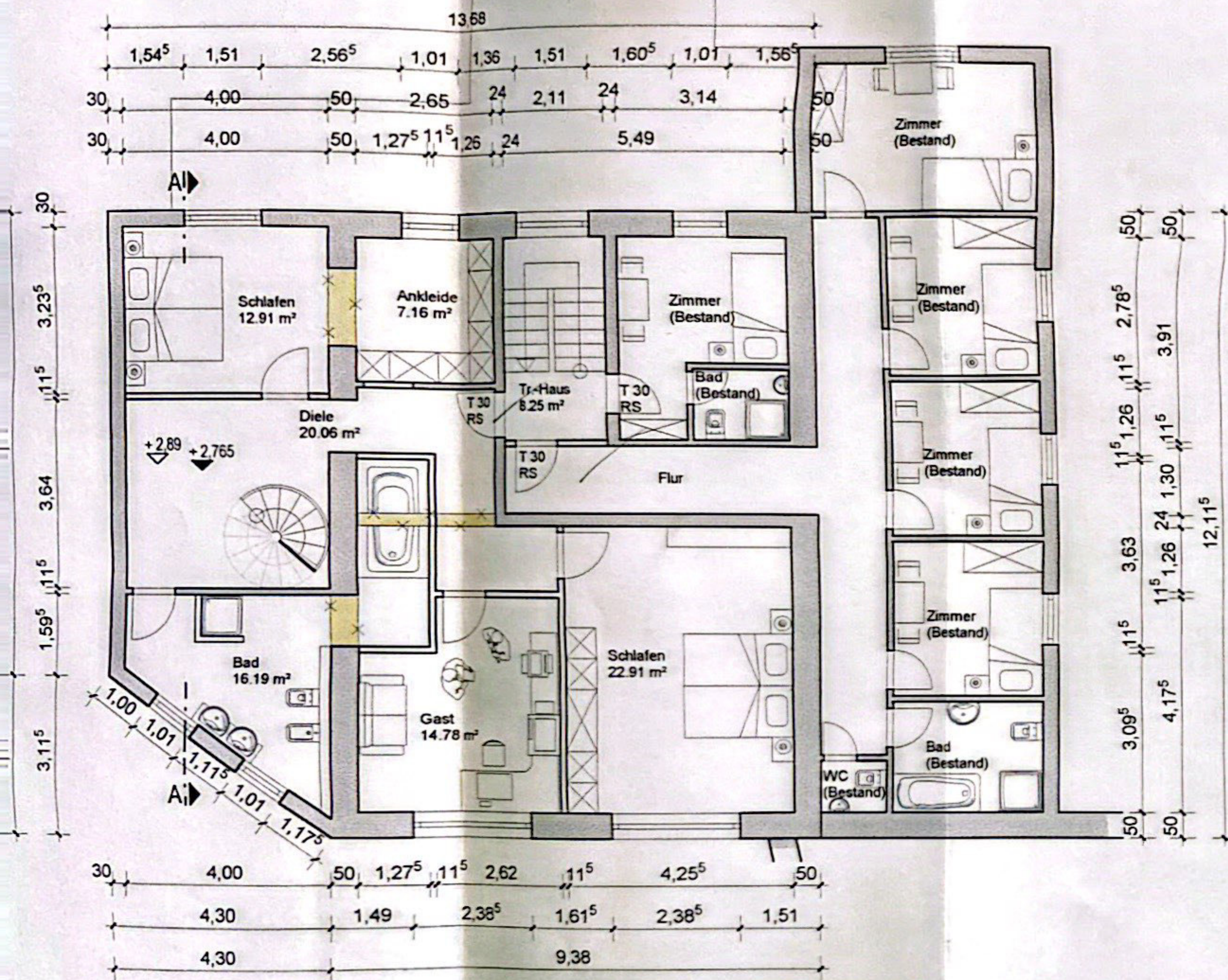
1. OBERGESCHOSS
