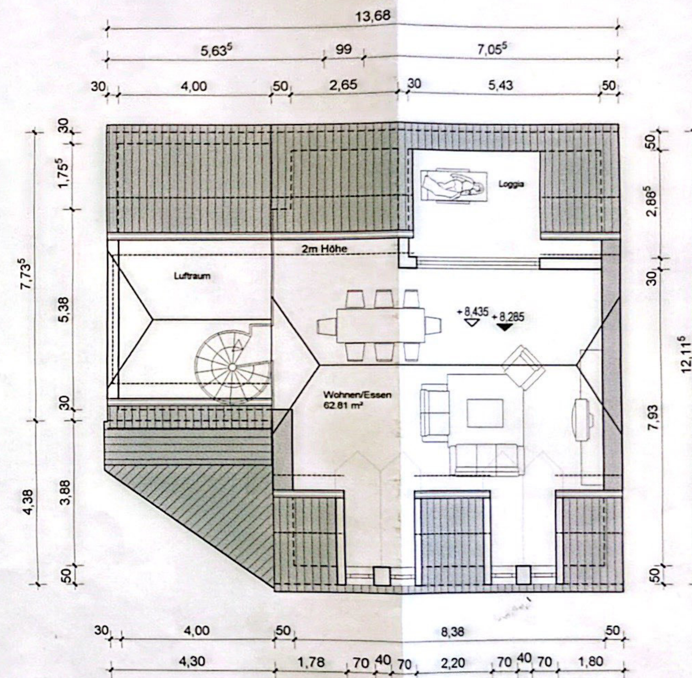
DACHGESCHOSS
