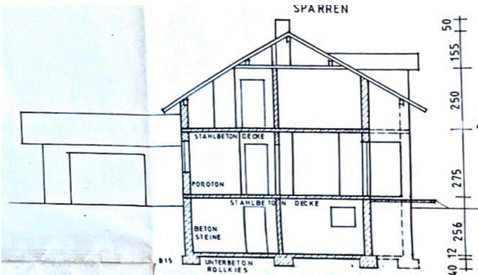
SCHNITT A.-A
