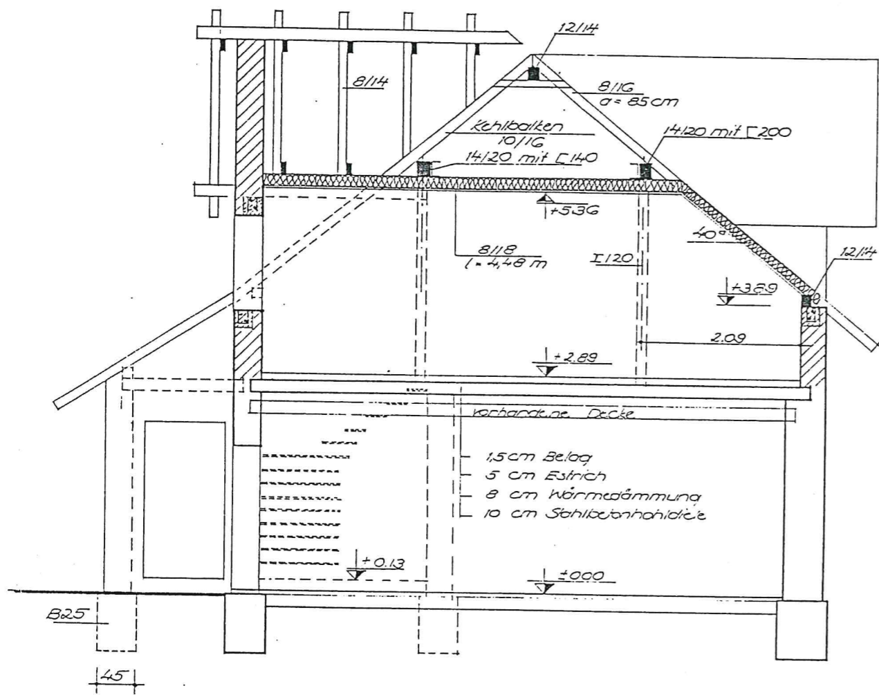
Schnitt A-A
