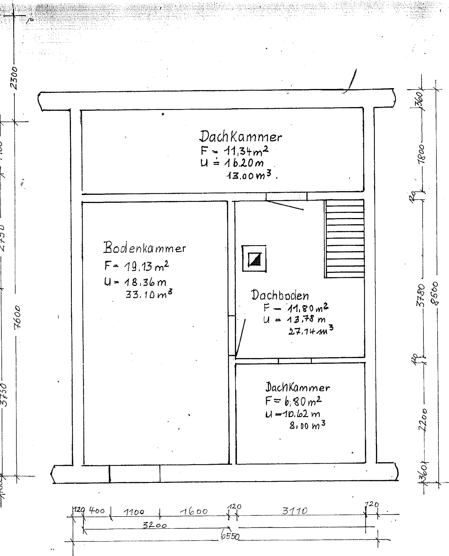
Dachgeschoss
