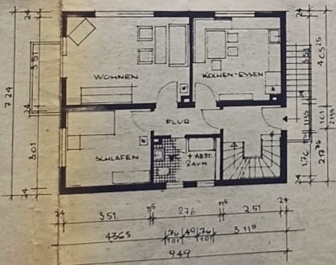
ERDGESCHOSS
