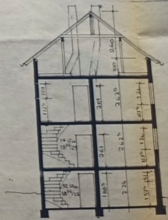
SCHNITT
