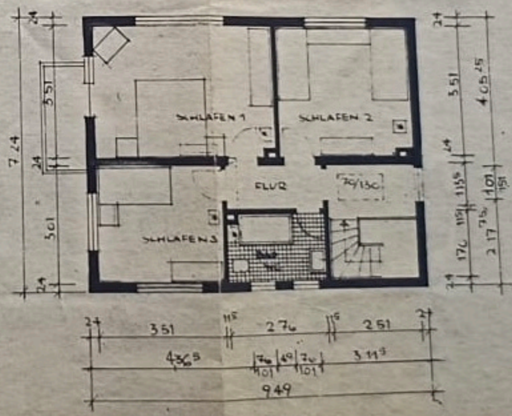
OBERGESCHOSS
