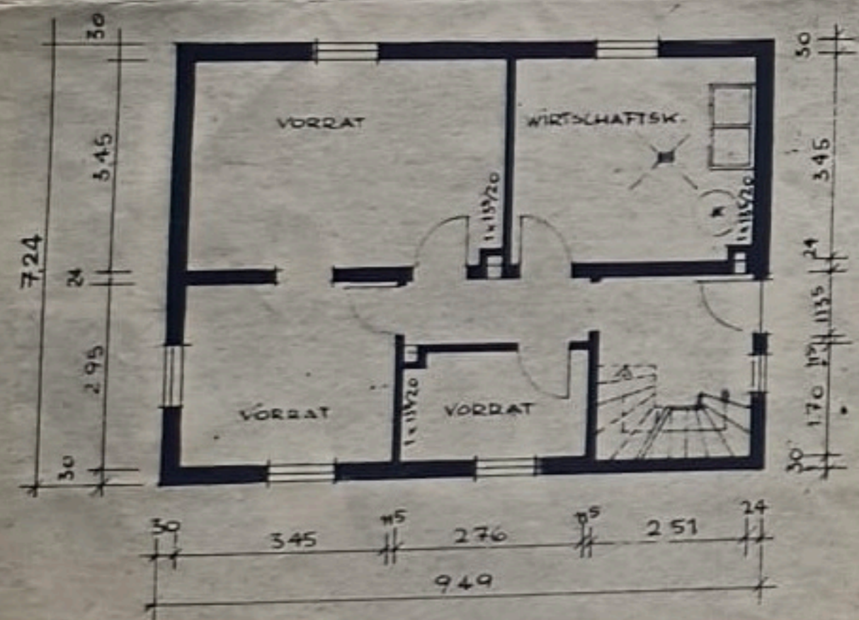
KELLERGESCHOSS
