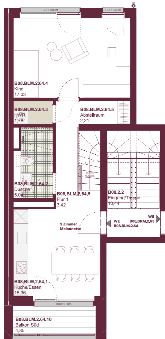
Grundriss 2. Obergeschoss M 1:100
