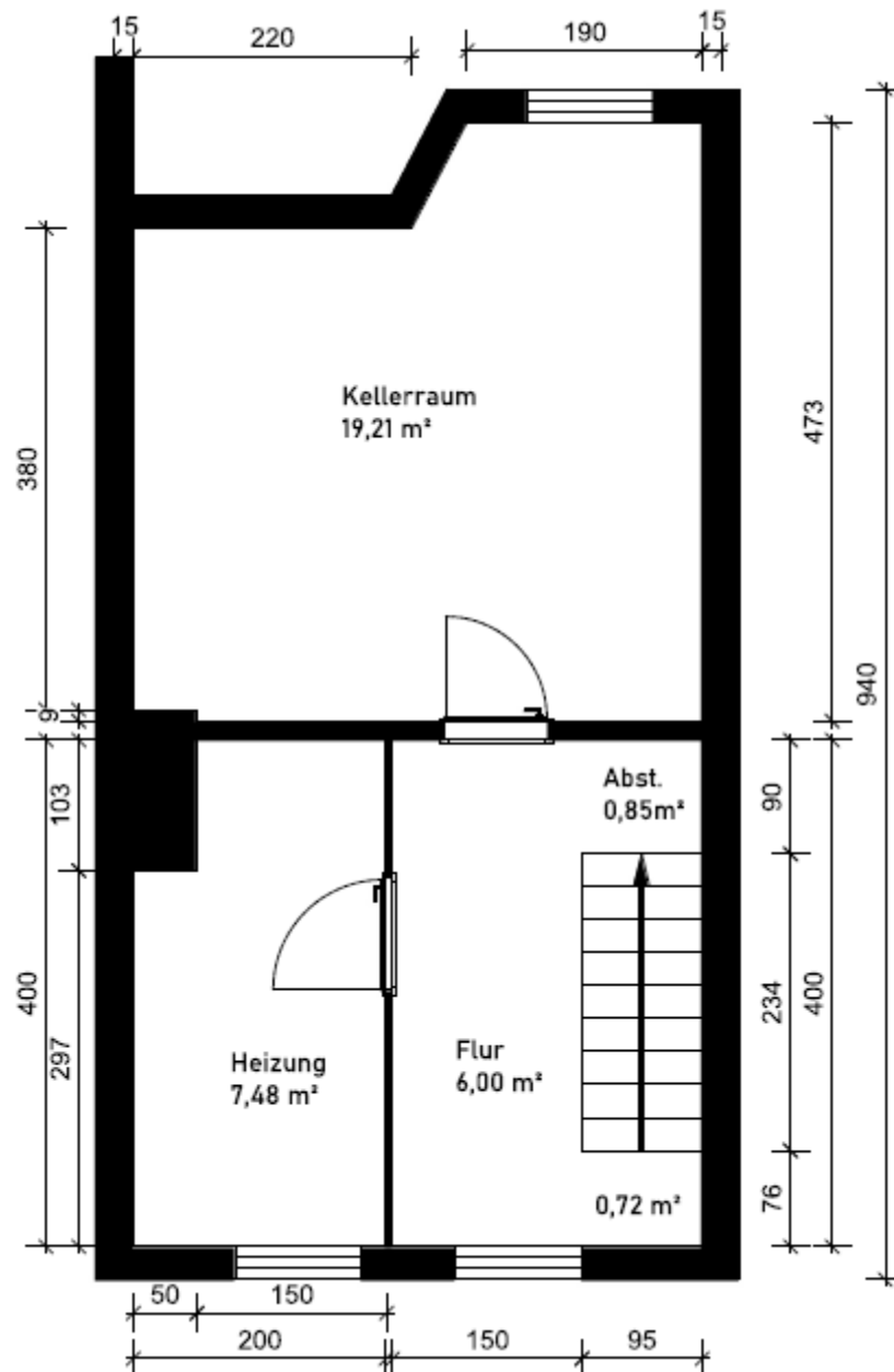
Grundriss Vollkeller
