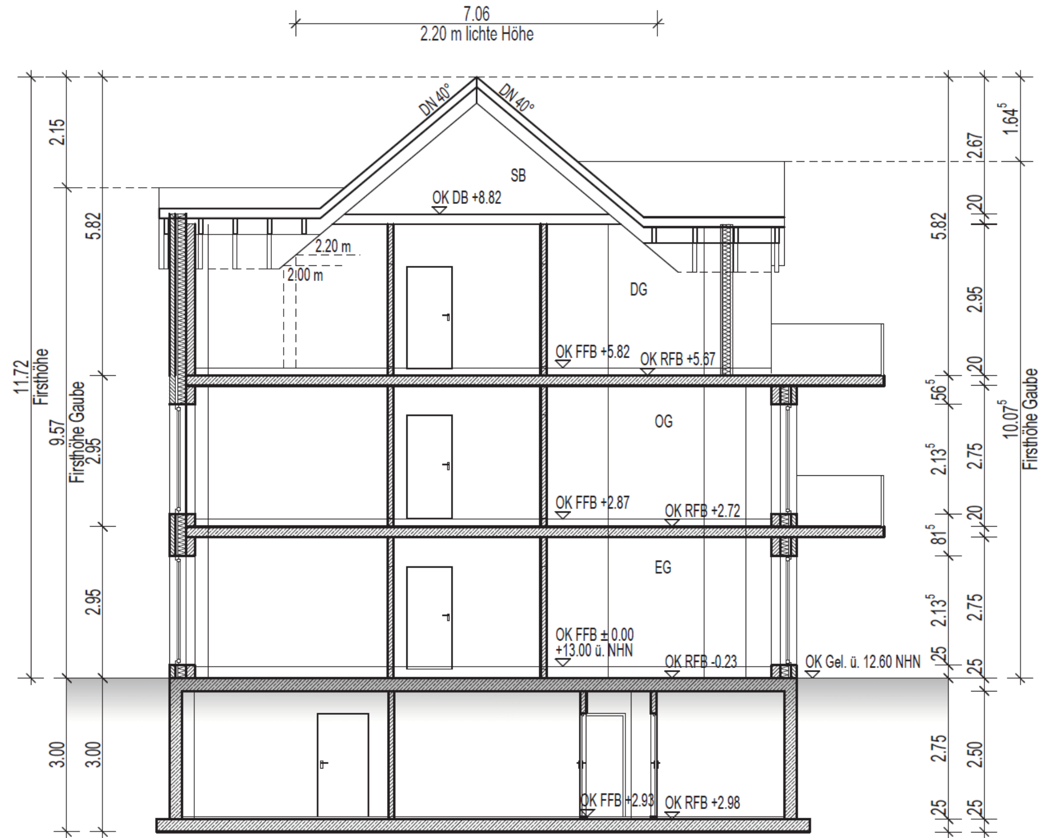
Schnitt B-B
