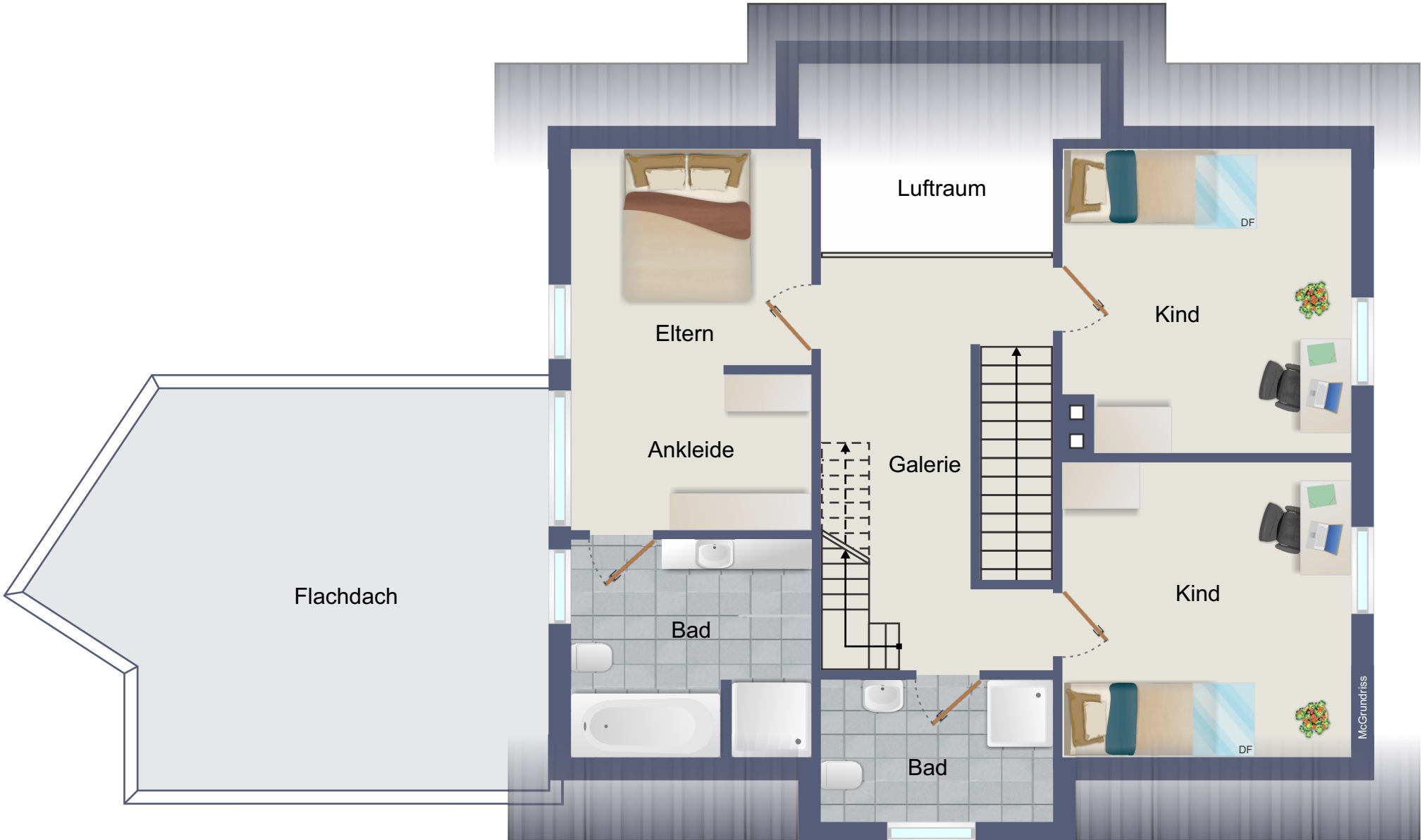
Dachgeschoss
