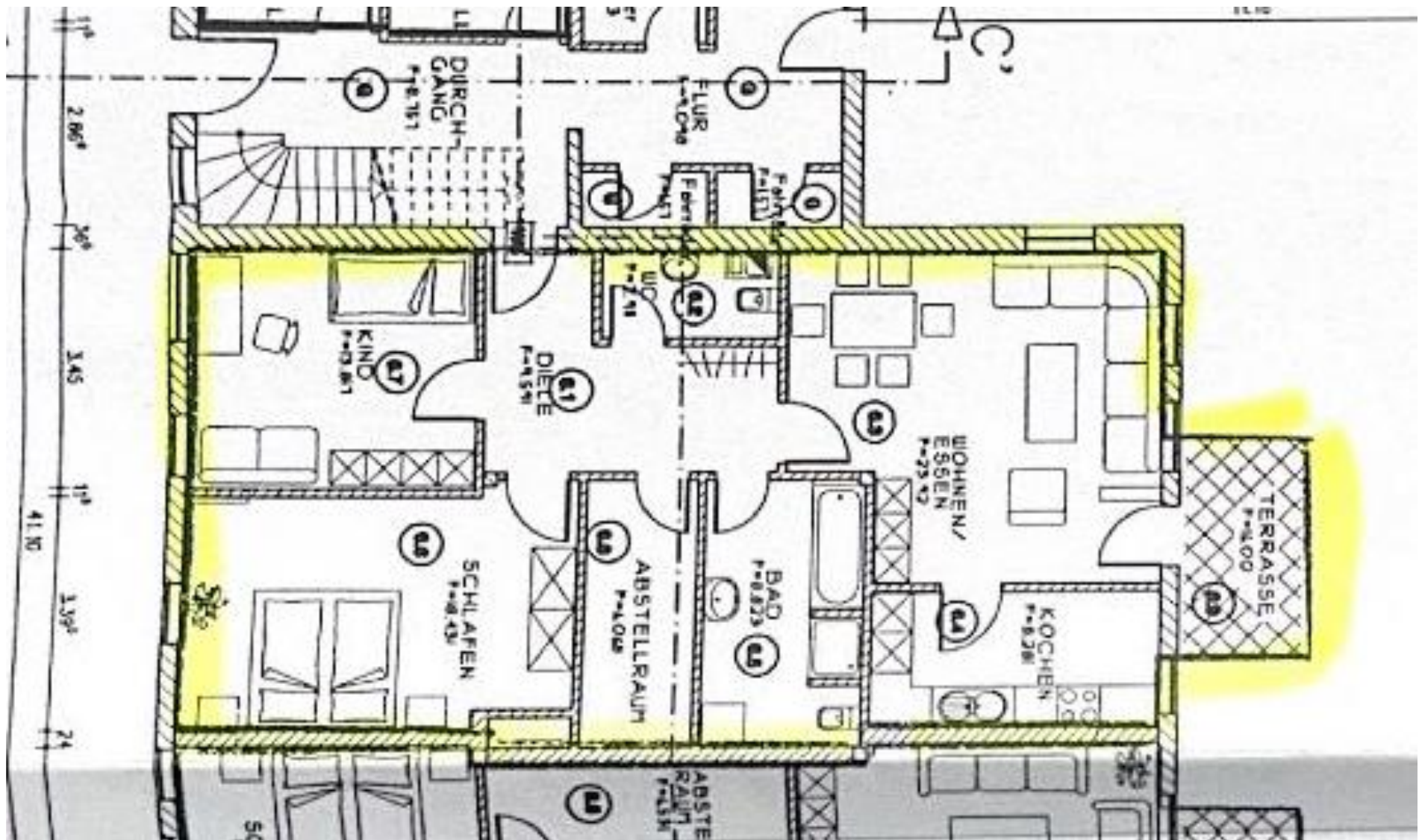
Grundriss Wohnung 6, Kreisstr. 24
