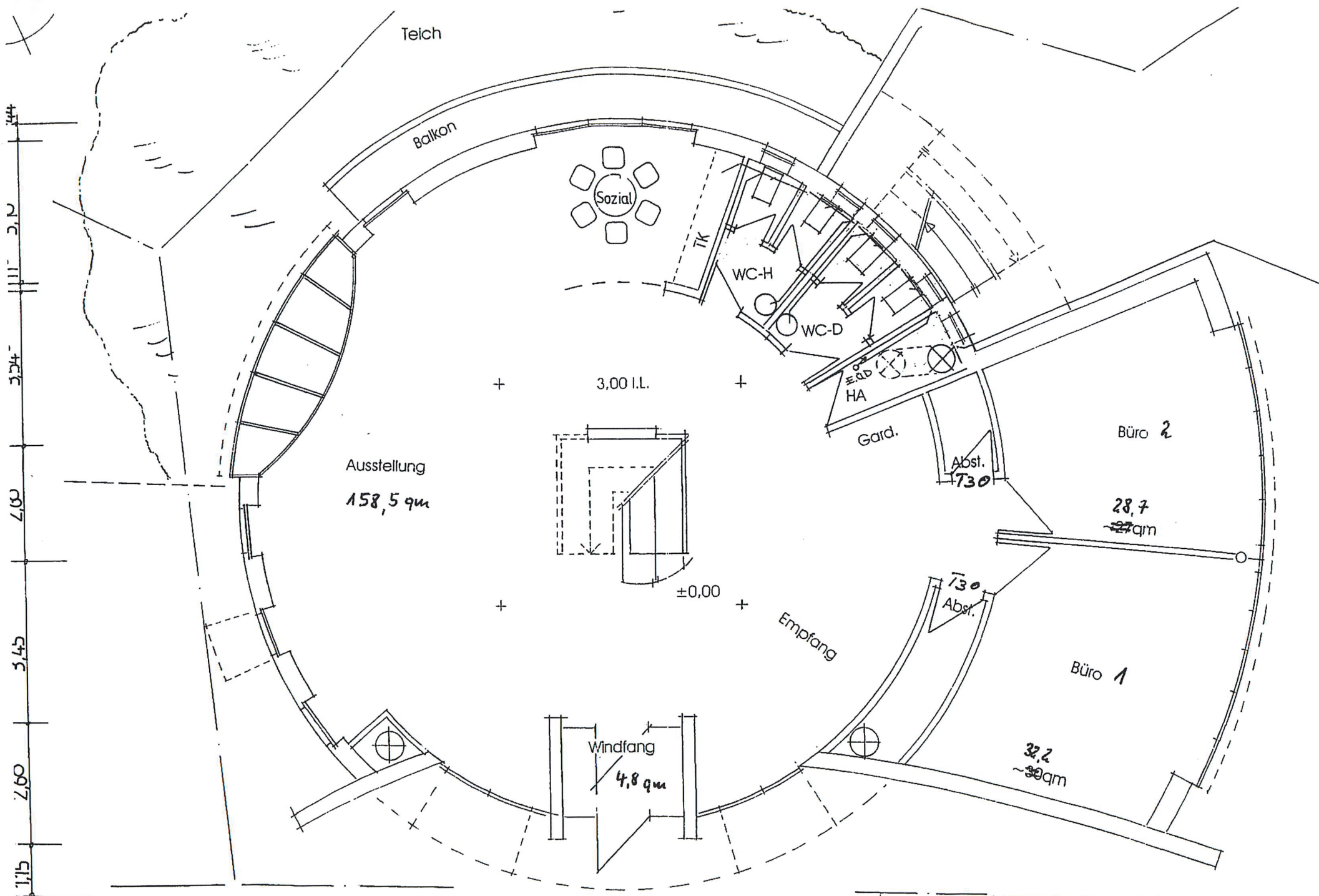
Erdgeschoss - Kontor-Haus
