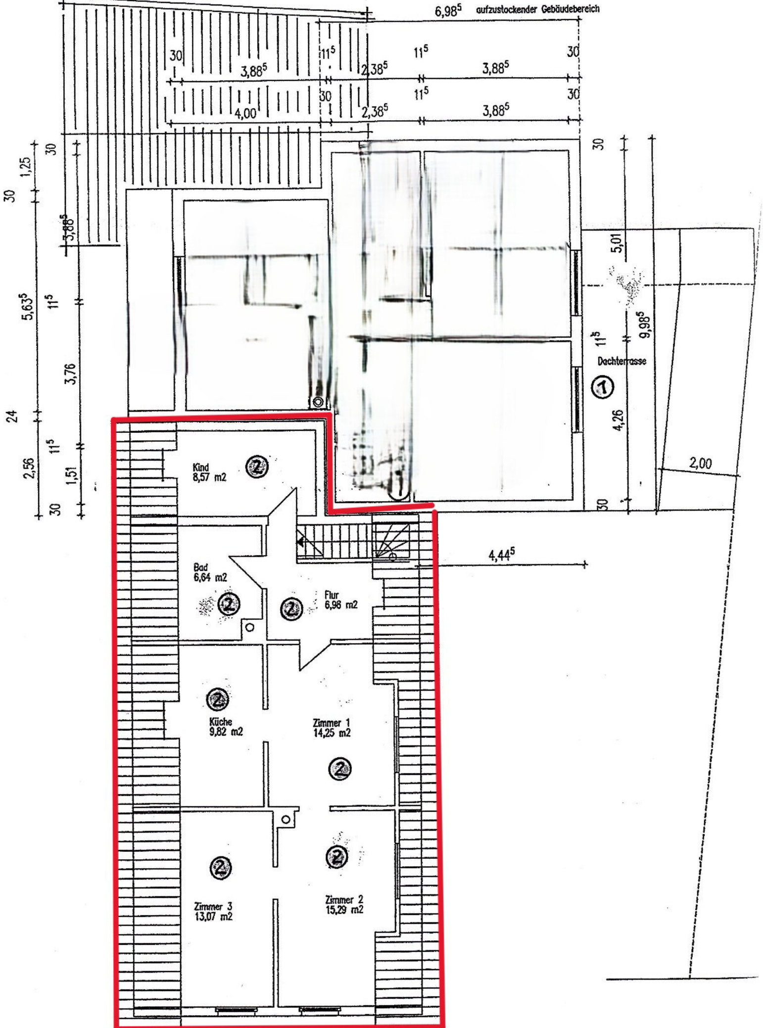
Grundriß Obergeschoß
