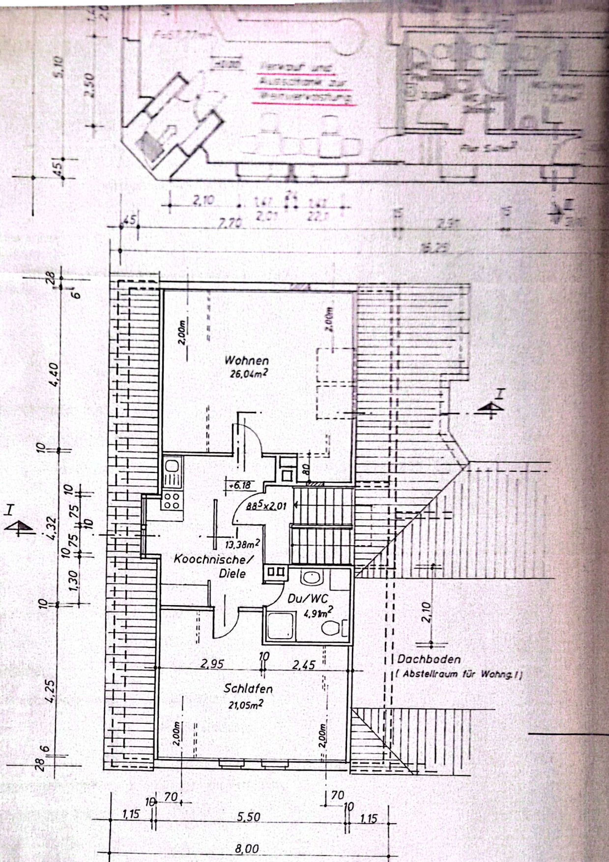
Grundriß DG 1:100
