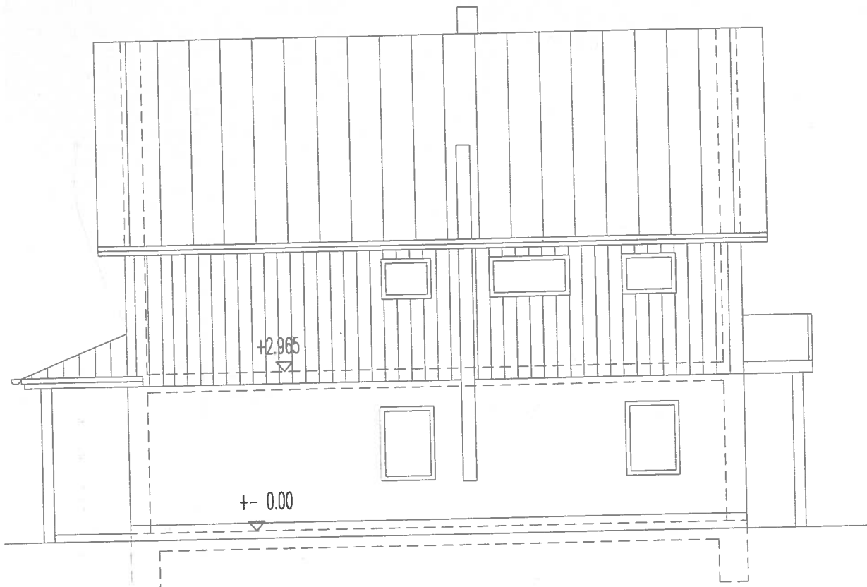
NORDANSICHT
