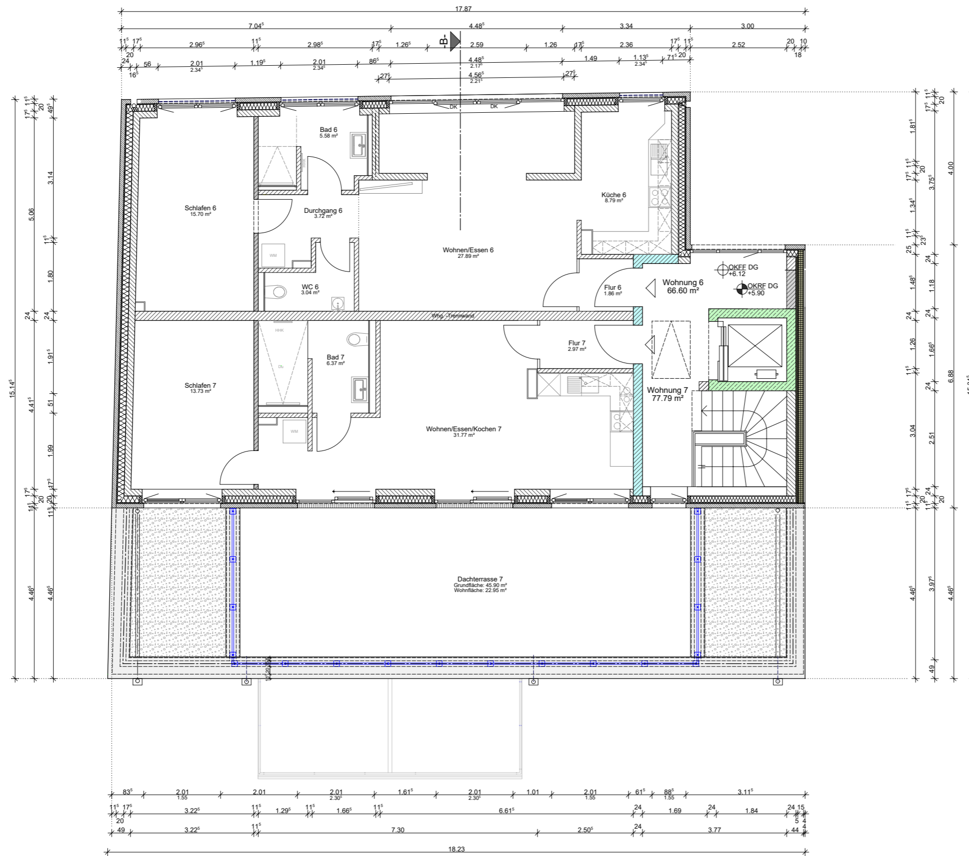
Grundriss Dachgeschoss
