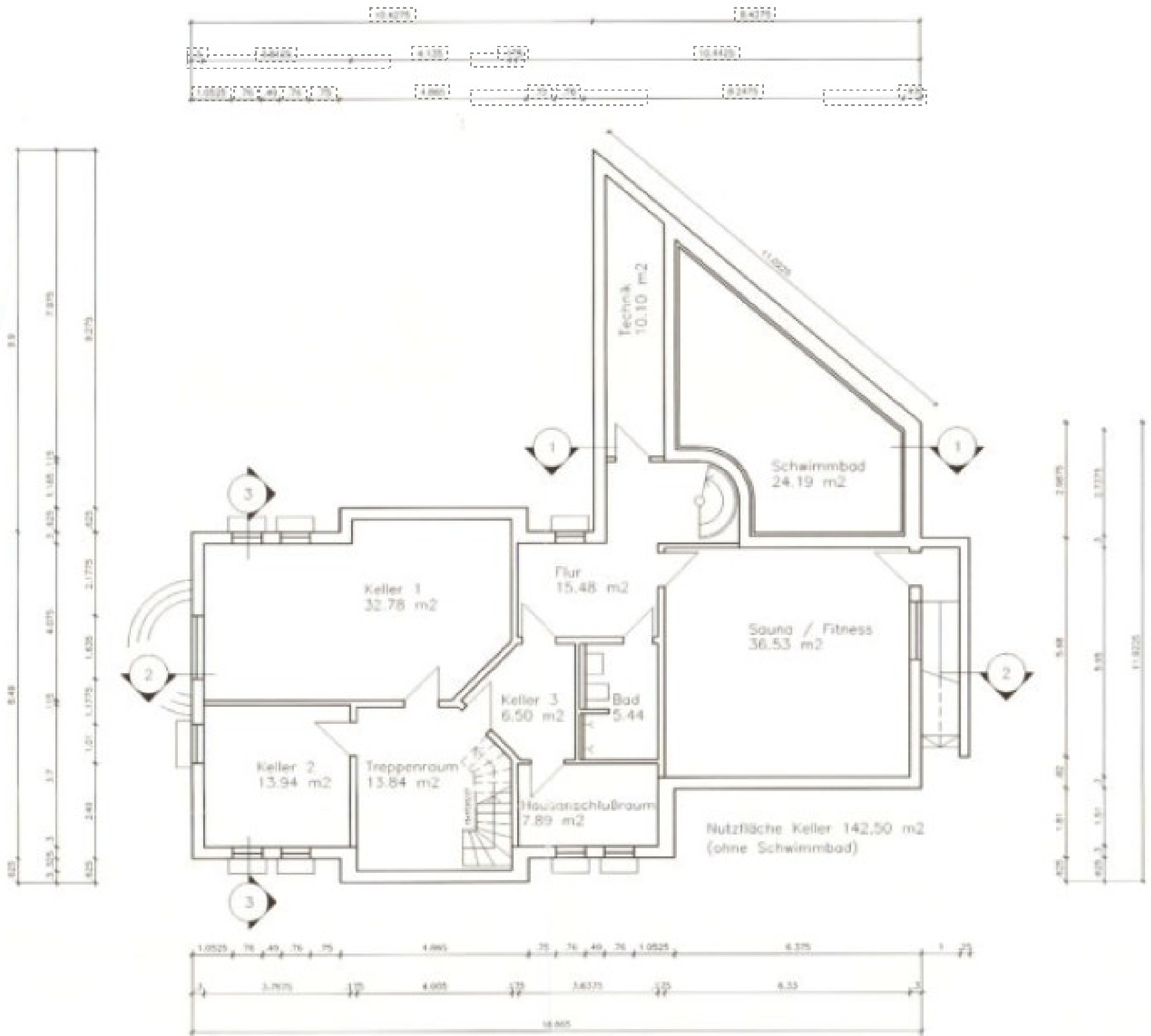
Grundriss Untergeschoss
