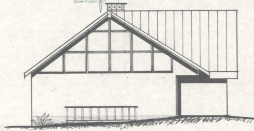
SÜDWESTANSICHT
