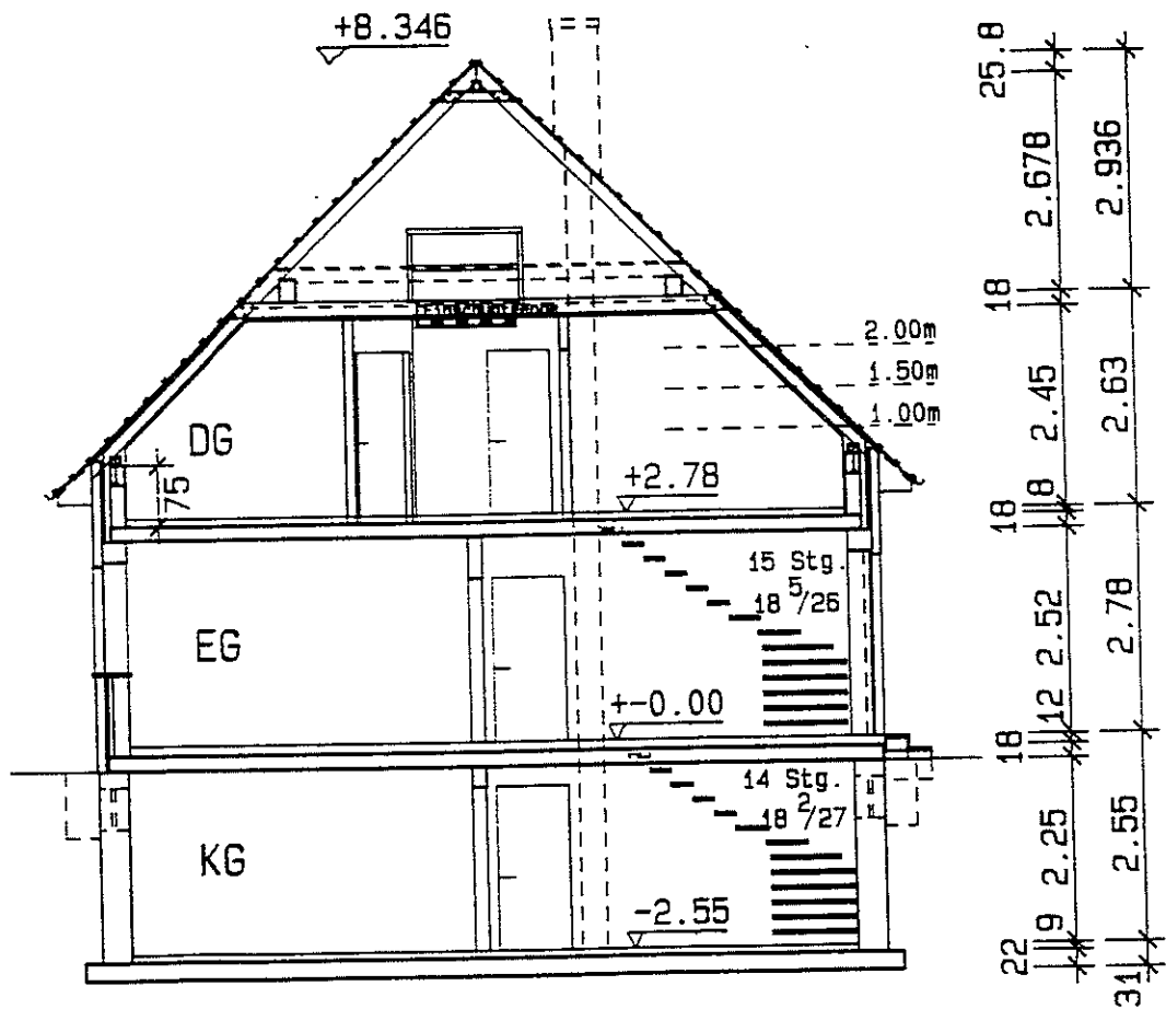
Schnitt A-A
