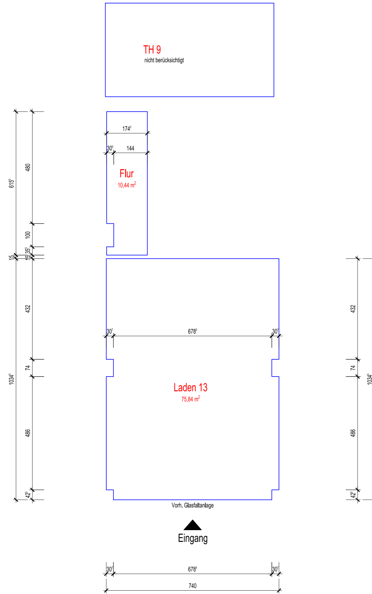
Laden 13 Grundriss Erdgeschoss Verkaufsraum und Flur
