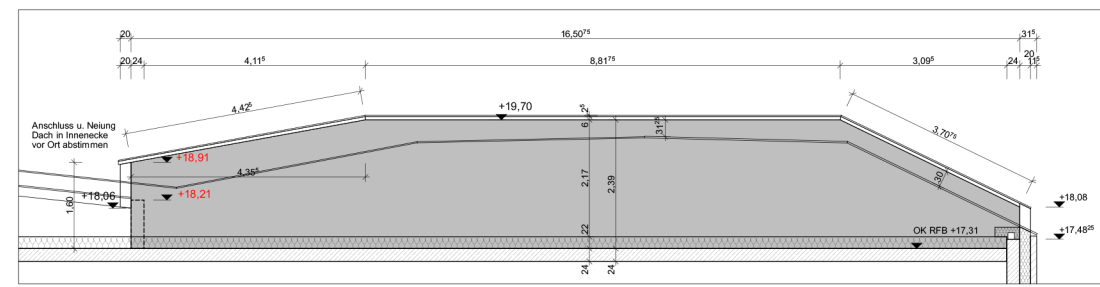
SCHNITTANSICHT 152.13 M. 1:50 BRANDWANDACHSE J
