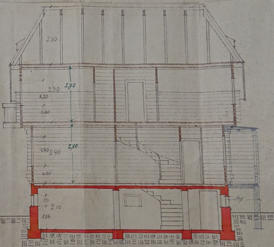
Längs-Schnitt.
