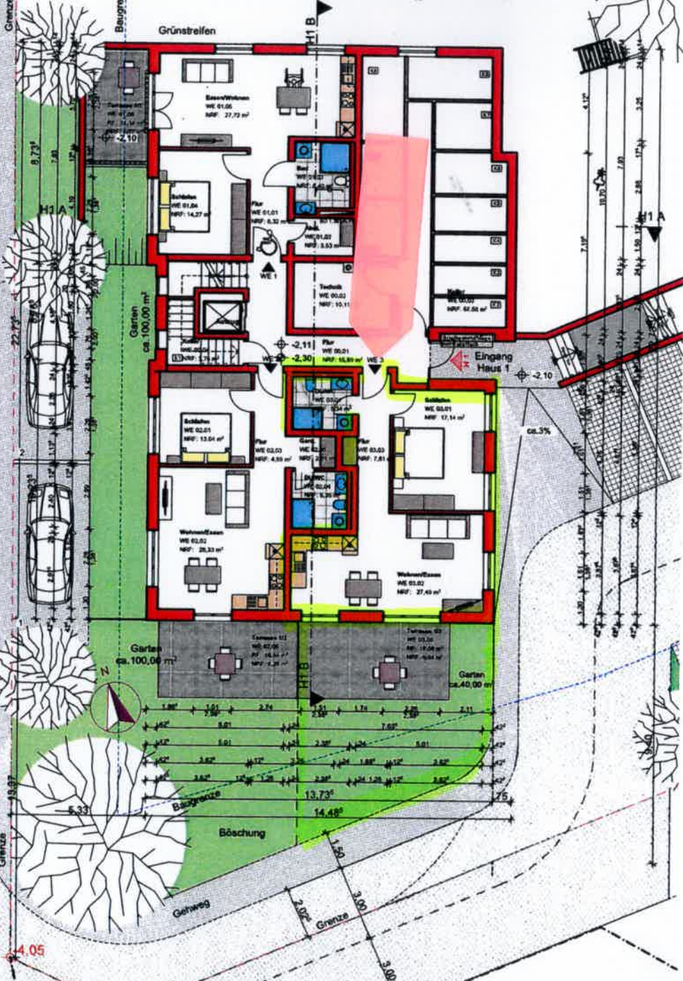
H1 Erdgeschoss M 1:100
