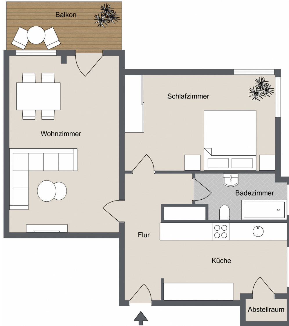
1. Etage
