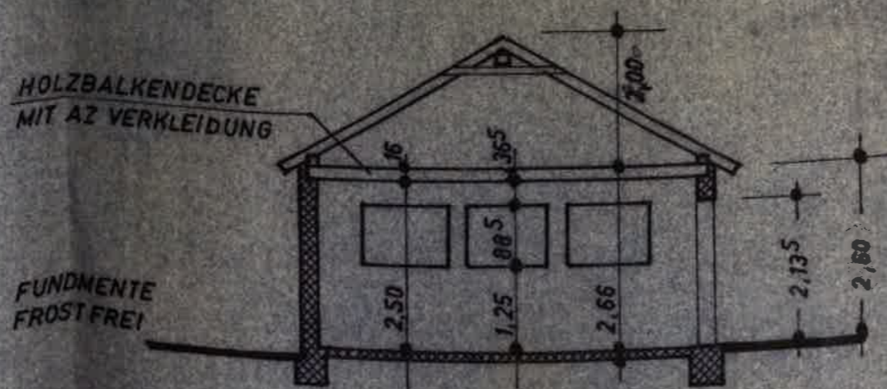
SCHNITT A-B
