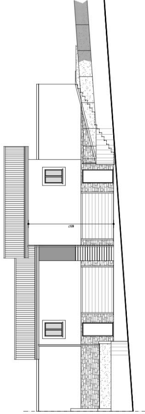
PROSPETTO NORD-EST
