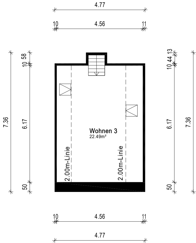
2. Dachgeschoss
