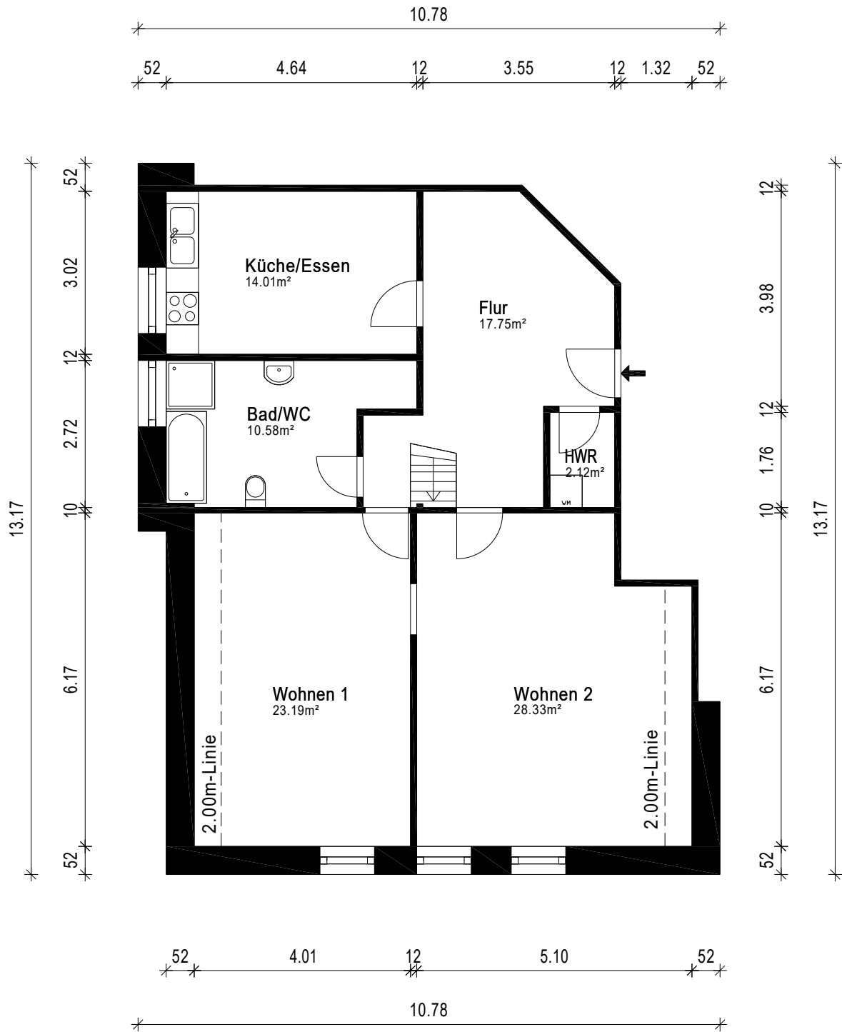
1. Dachgeschoss
