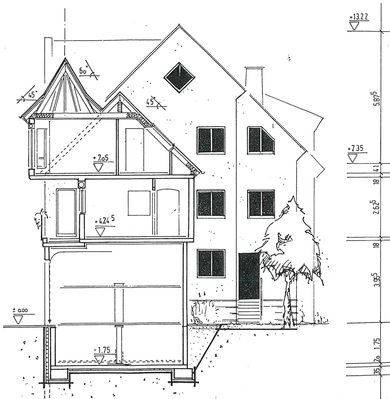
SCHNITT C-D / ANSICHT OST
