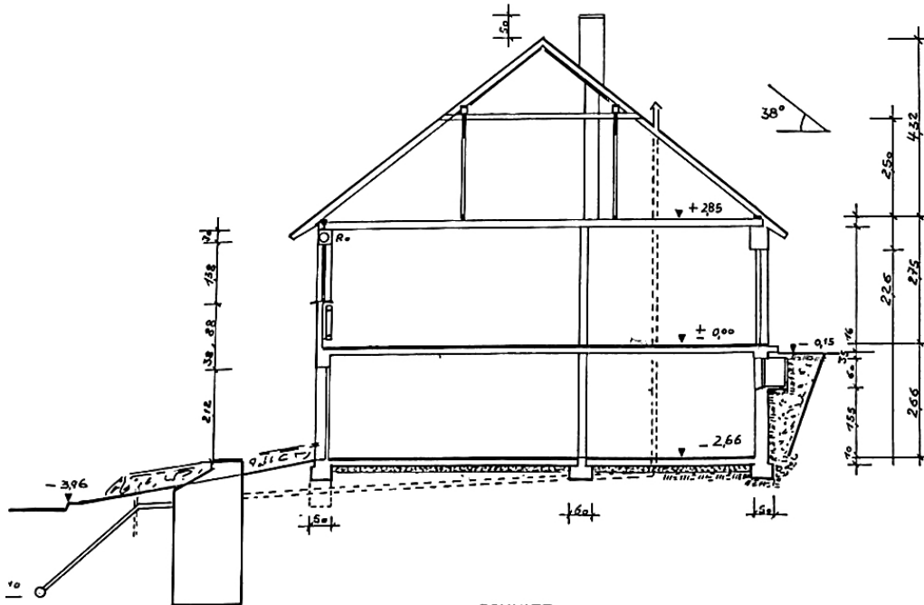
SCHNITT
