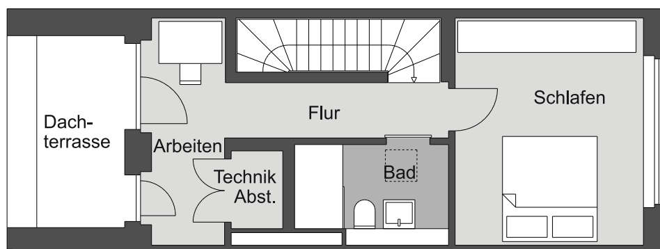
2. OG
