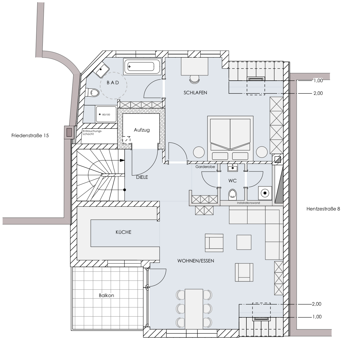
4. OBERGESCHOSS Wohnung 5- Ebene 1
