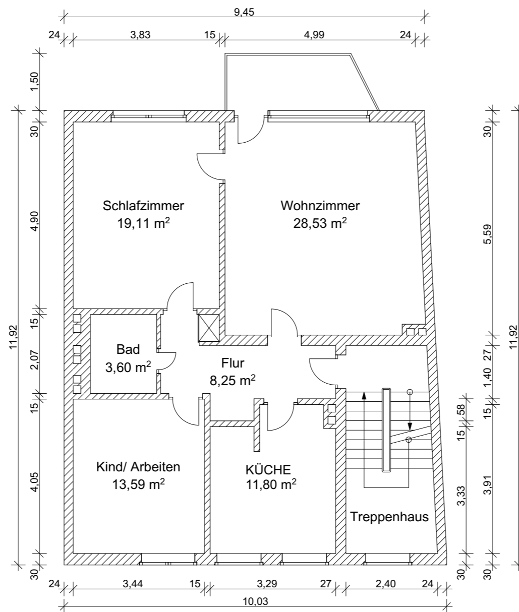
Grundriss OG3
