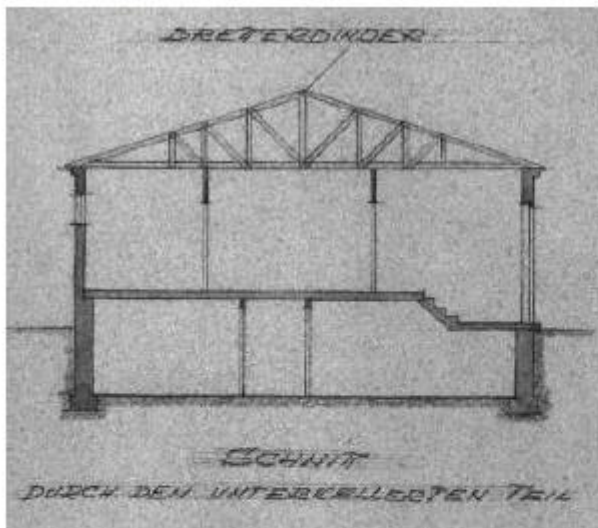
Gebäudeschnitt:
