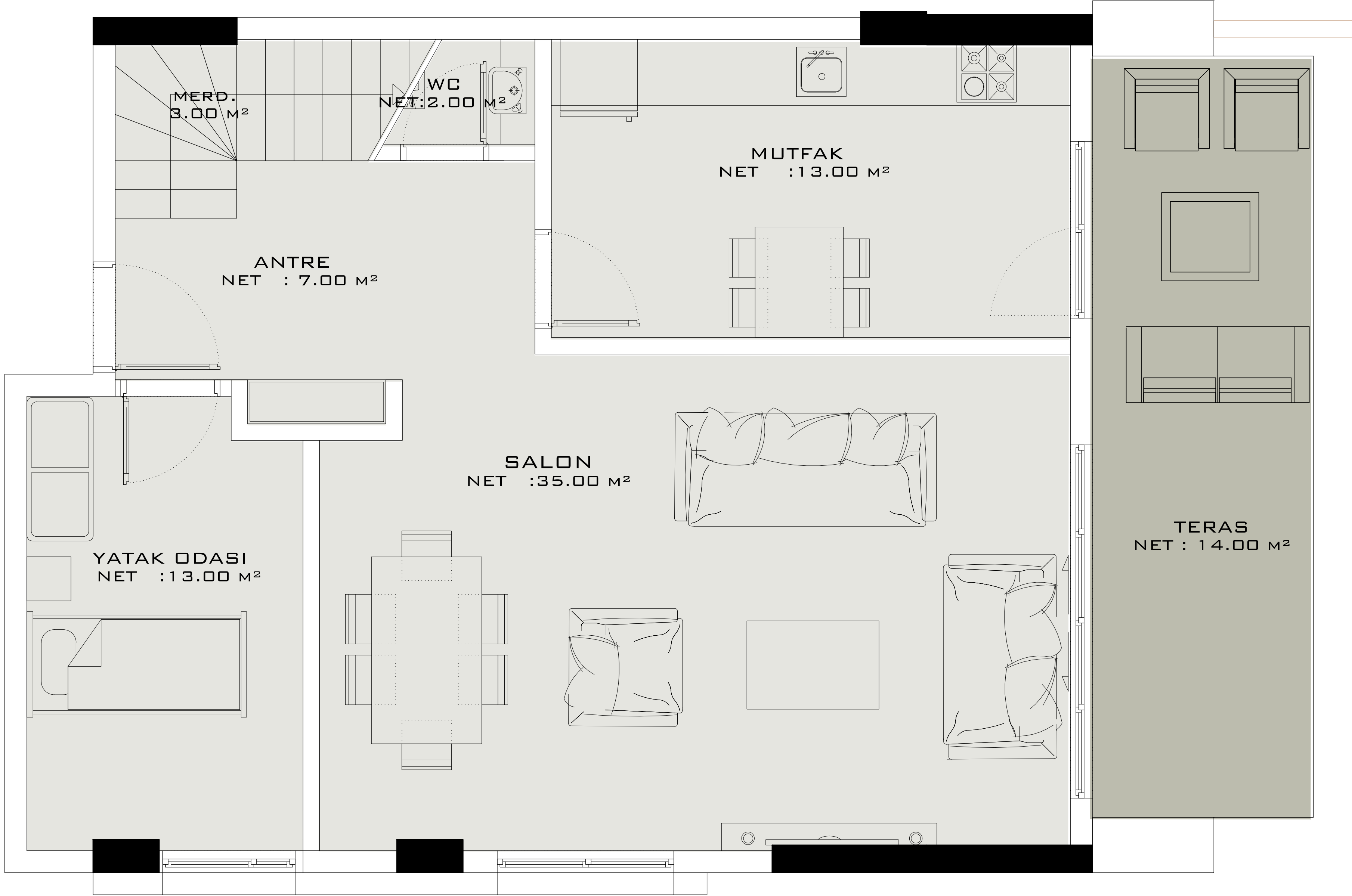
GİRİŞ KAT PLANI
