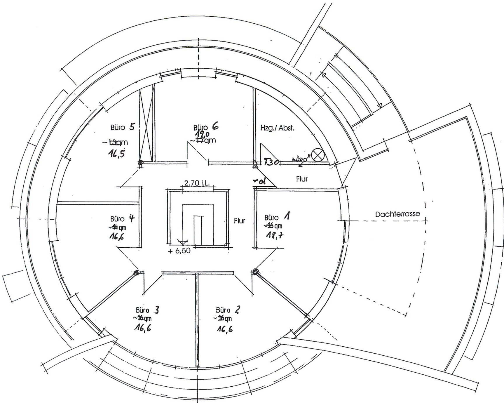
2. OG - Kontor-Haus
