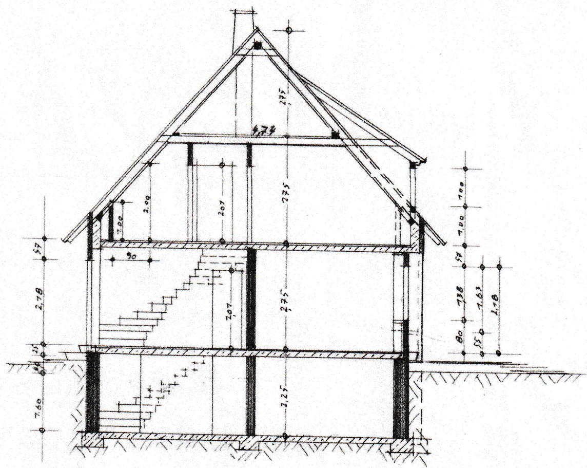
QUERSCHNITT
