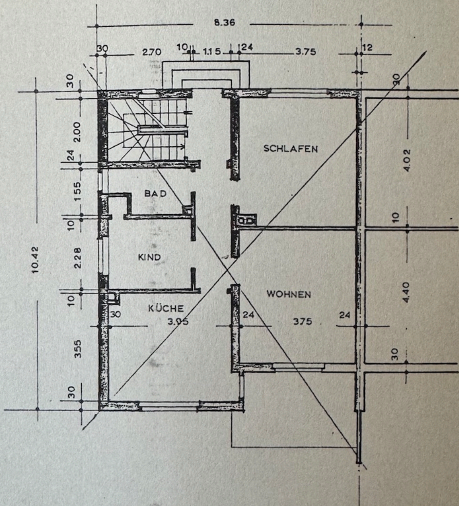
ERDGESCHOSS
