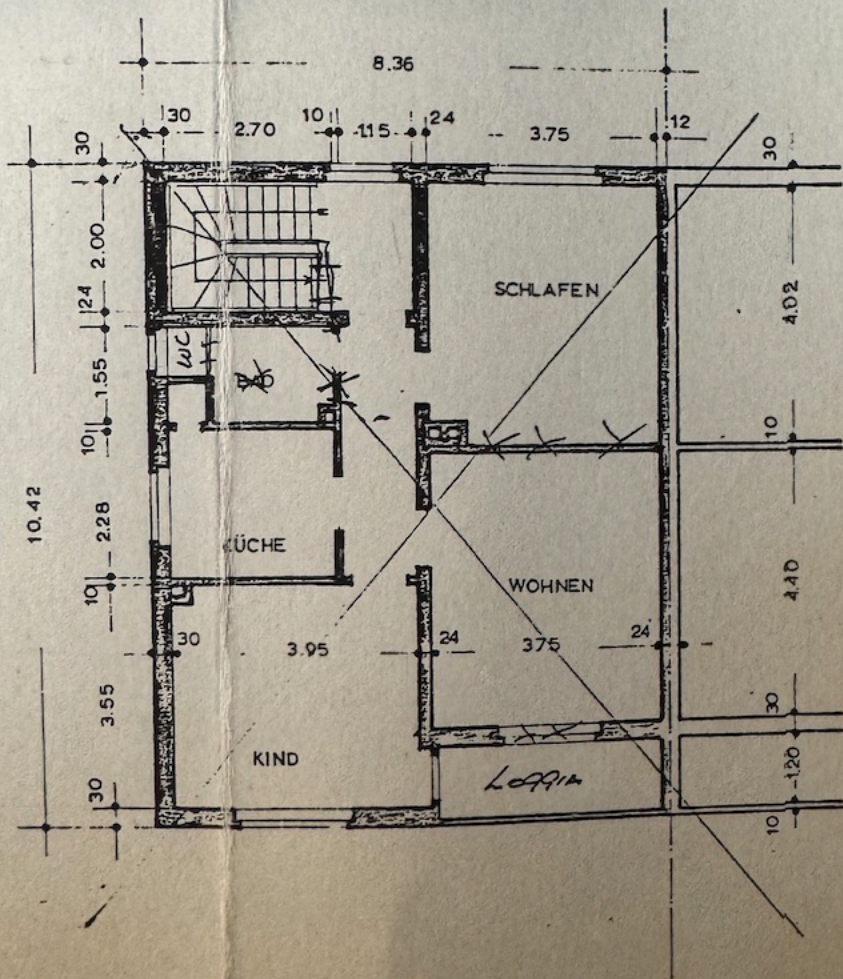
OBERGESCHOSS
