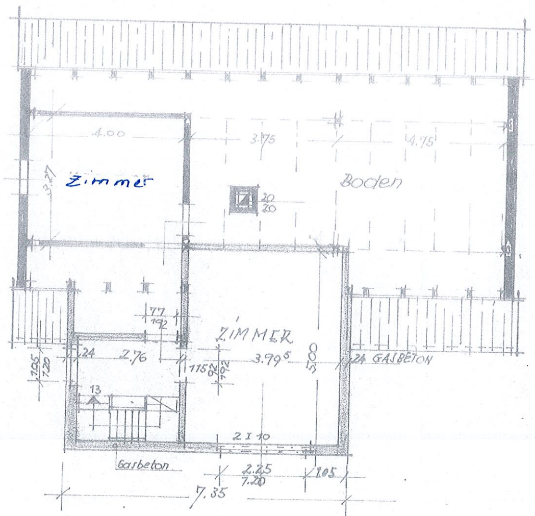
DACHGESCHOSS
