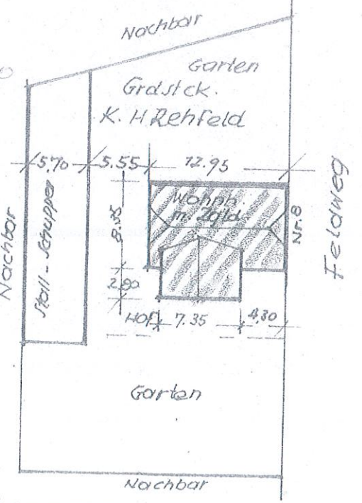
LAGEPLAN M. 1:500
