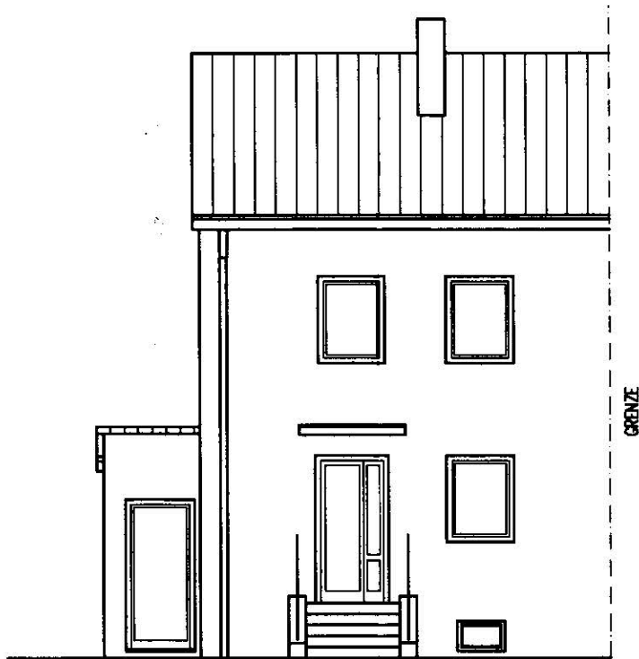
Ostansicht
