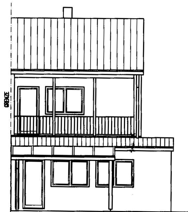
Westansicht
