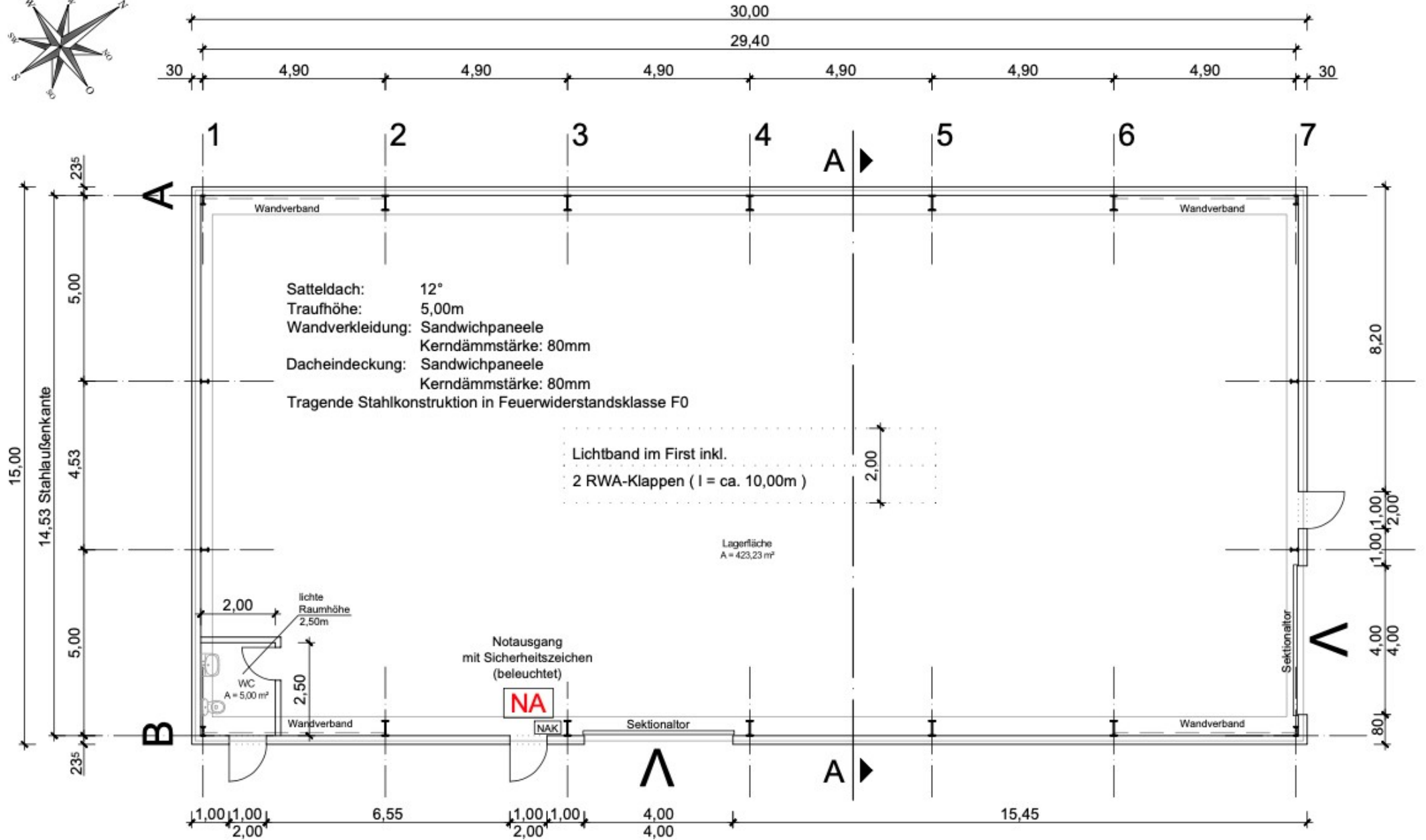
Grundriss
