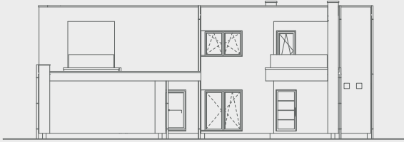
Ansicht vorne
