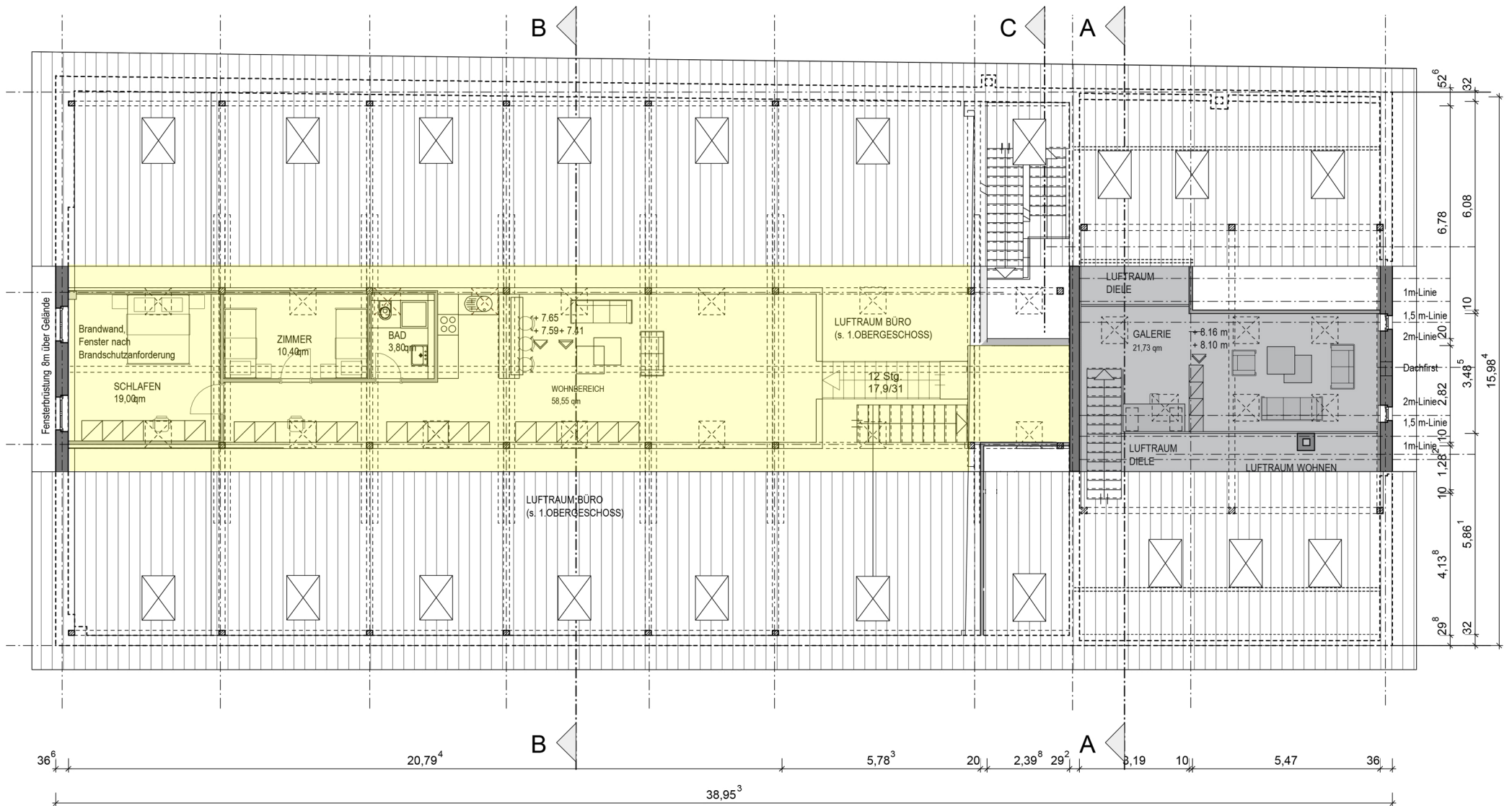
Grundriss Galerieschoss
